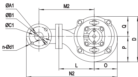
Размеры напорного патрубка насоса
