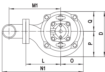
Фланцевое соединение с коленом
