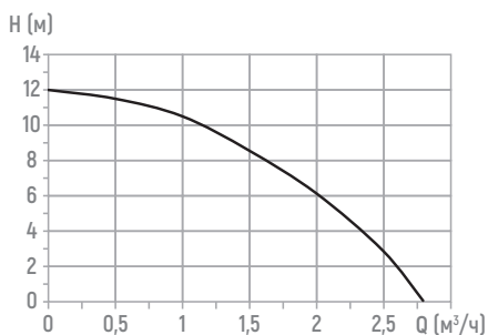
PROMO 15-12A
