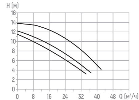
BASIC PRO 80-14SF, 3×380 В
