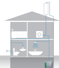
Применение в системе водоснабжения с накопительной ёмкостью
