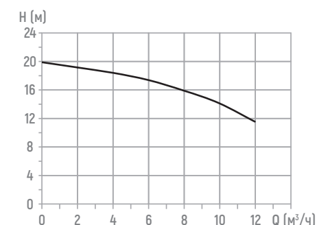
BASIC 25-20 230, 1 × 230 В
