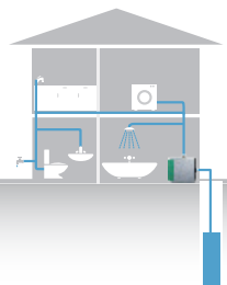
Применение в системе водоснабжения с колодезем
