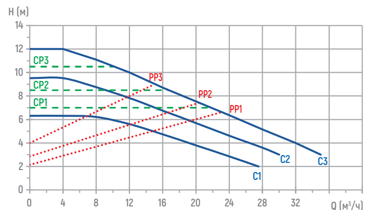
MEGA S 65-12F
