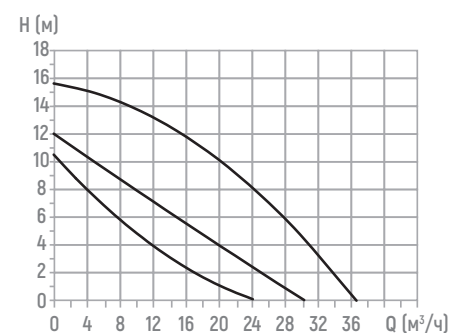
BASIC PRO 50-16SF, 1×230 В
