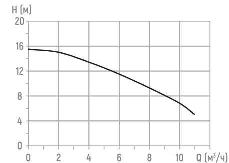
BASIC 25-16 230, 1 × 230 В
