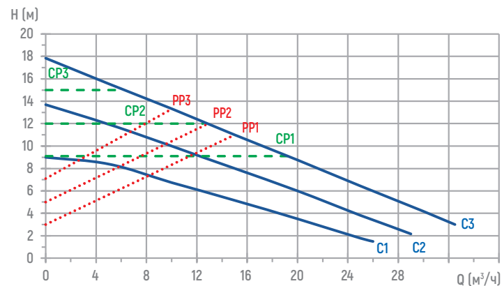
MEGA S 50-18F
